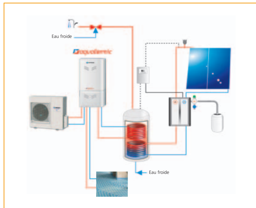
Schéma de fonctionnement du système Aquatermic
